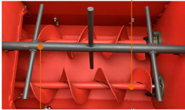
Componente del eje central antienredos
